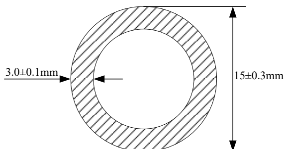
图 1 软管状标准截面示意图
